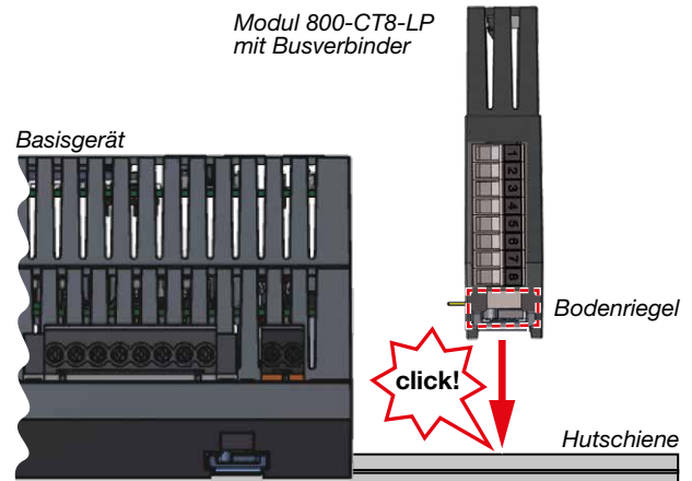
Abb.: Seitenansicht Basisgerät und Modul 800-CT8-LP
