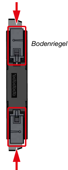
Abb.: Modul-Rückansicht
