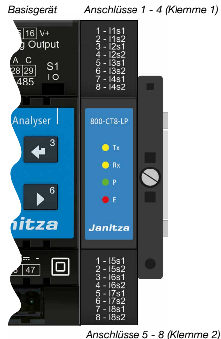
Abb. Anschlussvariante „Strommessung“ mit Modul 800-CT8-LP und Klemmenbelegung.
