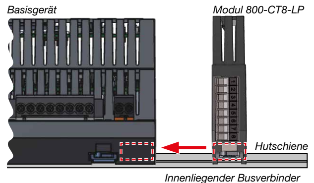
Abb.: Seitenansicht Basisgerät und Modul 800-CT8-LP
